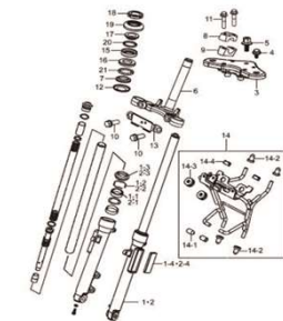
Fig.41 SUSPENSÃO DIANTEIRA (P05-C400-0006)
