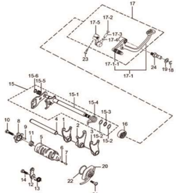
Fig.17 PEDAL DE CAMBIO (P05-C160-0003)
