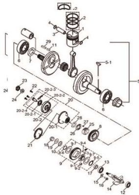
Fig.5 VIRABREQUIM DO MOTOR (P05-C050-0007)
