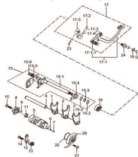
Fig.17 PEDAL DE CAMBIO (P05-C160-0003)
