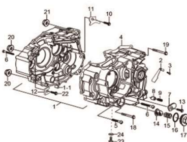
Fig.3 CARCAÇA DO MOTOR (P05-C030-0010)
