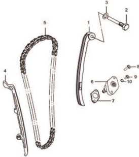
Fig.8 CORRENTE DE COMANDO (P05-C080-0003)
