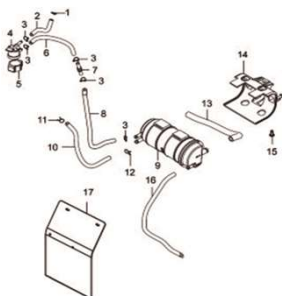
Fig.10 VALVULA DE EVAPORAÇÃO (P05-C098-0004)
