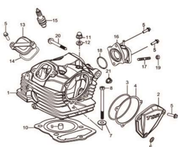
Fig.1 CABEÇOTE DO MOTOR (P05-C010-0011)
