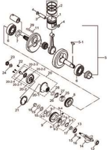
Fig.5 VIRABREQUIM DO MOTOR (P05-C050-0007)
