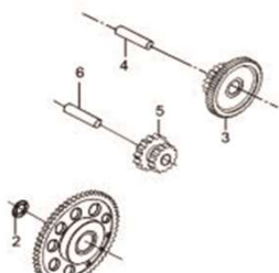
Fig.6 ENGRENAGEM DE PARTIDA (P05-C060-0001)
