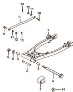
Fig.46 BALANÇA TRASEIRA (P05-C440-0002)
