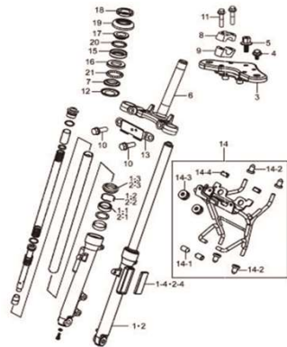
Fig.41 SUSPENSÃO DIANTEIRA (P05-C400-0006)
