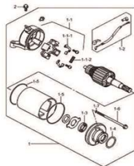
Fig.18 MOTOR DE PARTIDA (P05-C170-0002)
