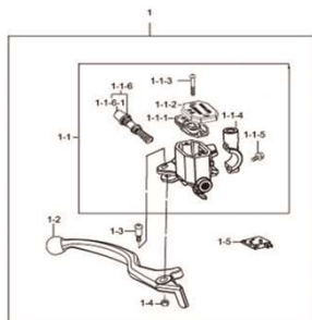
Fig.44 CILINDRO DE FREIO DIANTEIRO (P05-C430-0002)
