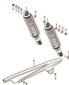
Fig.47 AMORTEDEDOR TRASEIRO (P05-C450-0003)
