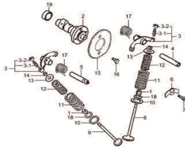
Fig.7 COMANDO DE VALVULAS(P05-C070-0006)
